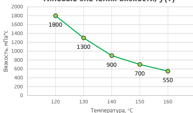
Типовые значения вязкости, f(T)
