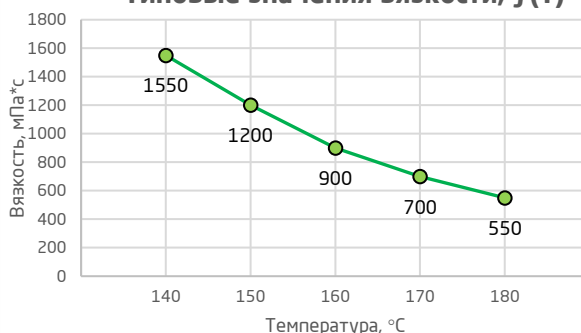
Типовые значения вязкости, f(T)
