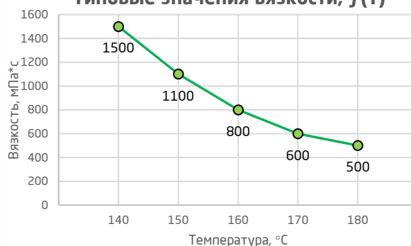
Типовые значения вязкости, f(T)
