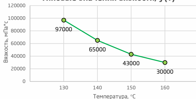
Типовые значения вязкости, f(T)
